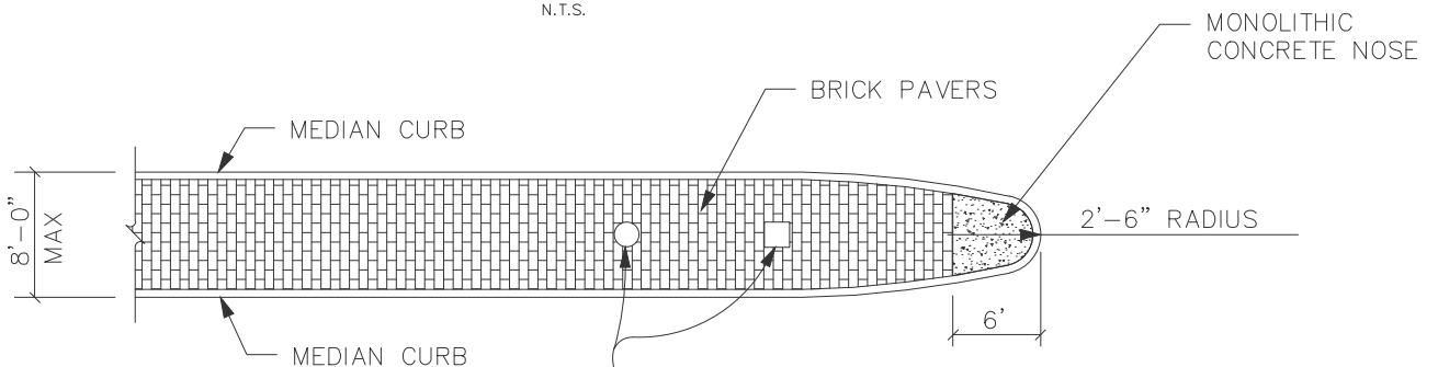
MEDIAN NOSE TYPE "B" N.T.S.
