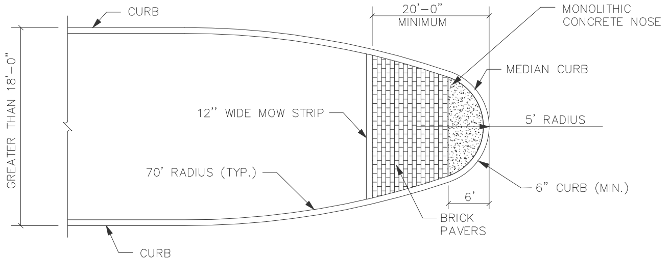
MEDIAN NOSE TYPE "C" N.T.S.
