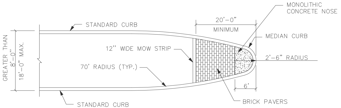
MEDIAN NOSE TYPE "C" N.T.S.
